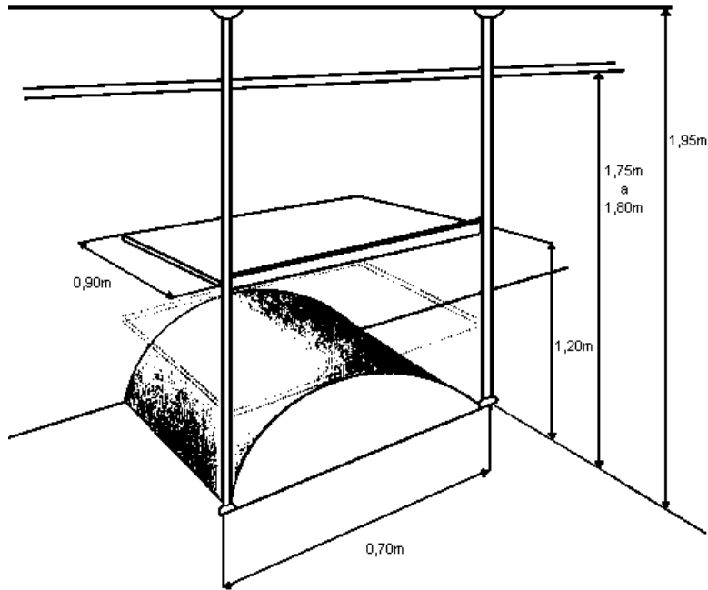
FIGURA 5 AREA DE CARGA
